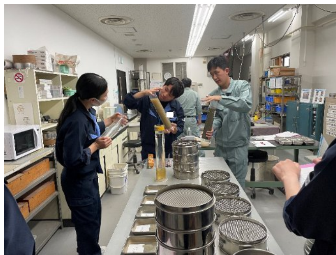
室内土質試験の研修②
